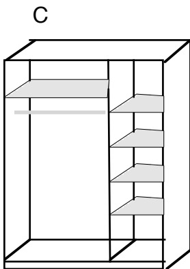
C: Korpus für 3Türen mit Mittelwand 5 Böden 1 Stange
